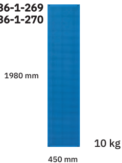
FYRKANTIGA HÅL / SQUARE HOLES 10x10 mm CC mått 20 mm
