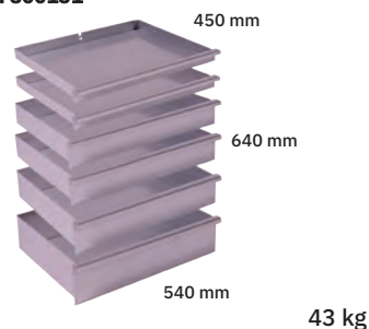
LÅDSATS 6 / DRAWER SET 6 Article no. 800131
